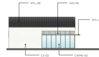
ELEVATION 3
