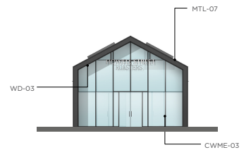
ELEVATION 4
