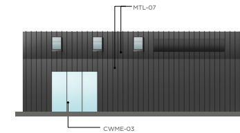
ELEVATION 3
