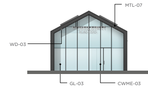
ELEVATION 2
