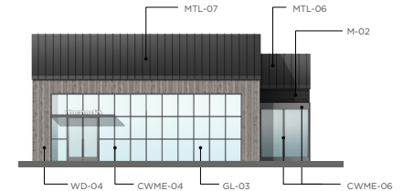
ELEVATION 4
