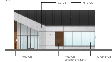
ELEVATION 3
